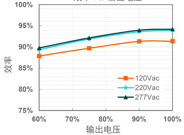
EAM-150S210DB( I_o=2100mA )
