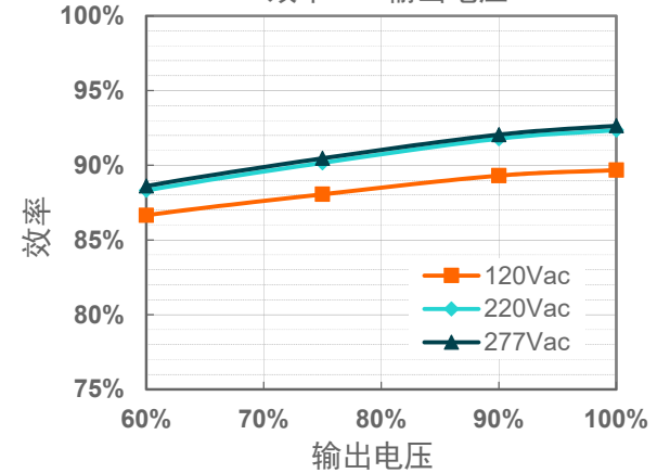
EAM-150S420DB( I_o=4200mA )
