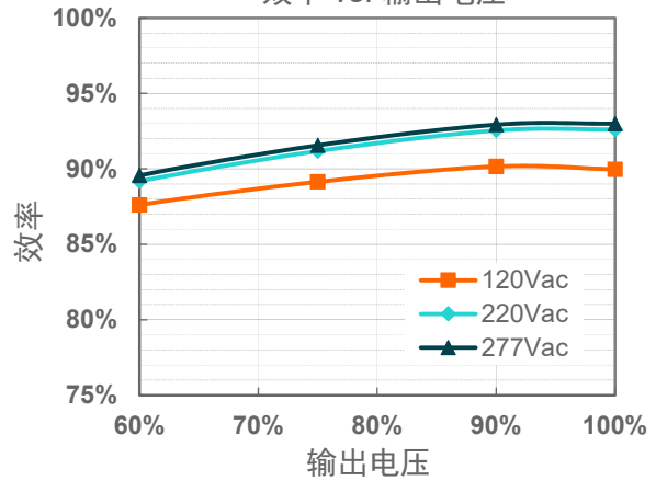
EAM-150S420DB( I_o=4200mA )
