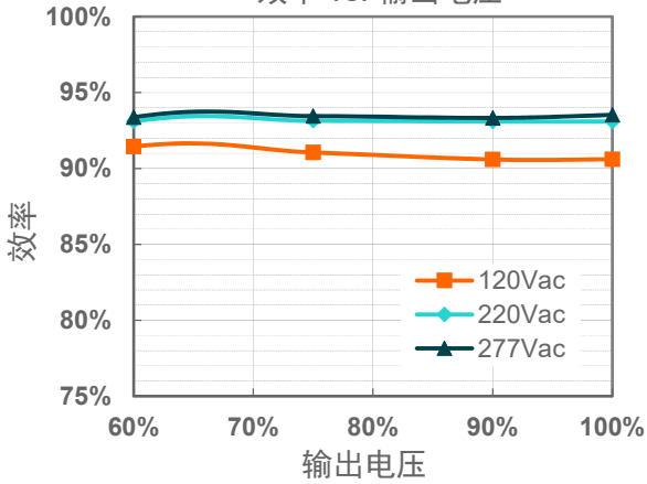
EAM-150S210DB( I_o=1400mA )
