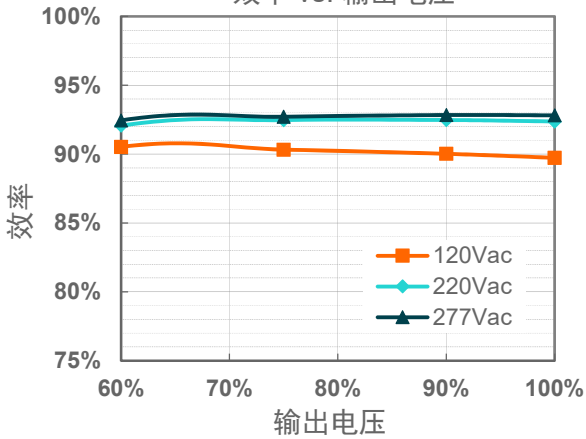
EAM-150S420DB( I_o=2800mA )
