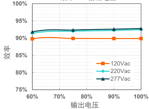
EAM-150S420DB( I_o=2800mA )
