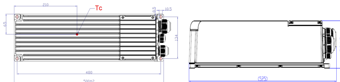
驱动器结构图和 Tc 的位置
